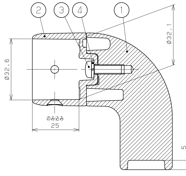
A-A断面図 (S=1/1)
